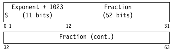
Figure 19-5. BFP Long Format (8 bytes)
