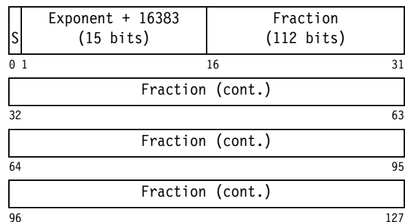
Figure 19-6. BFP Extended Format (16 bytes)
