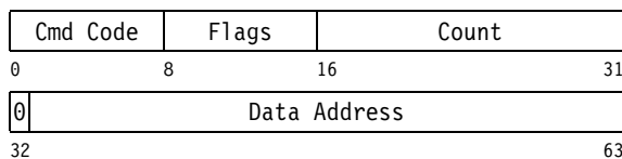
Format-1 CCW
