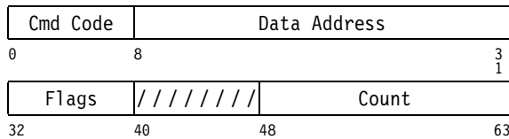
Format-0 CCW
